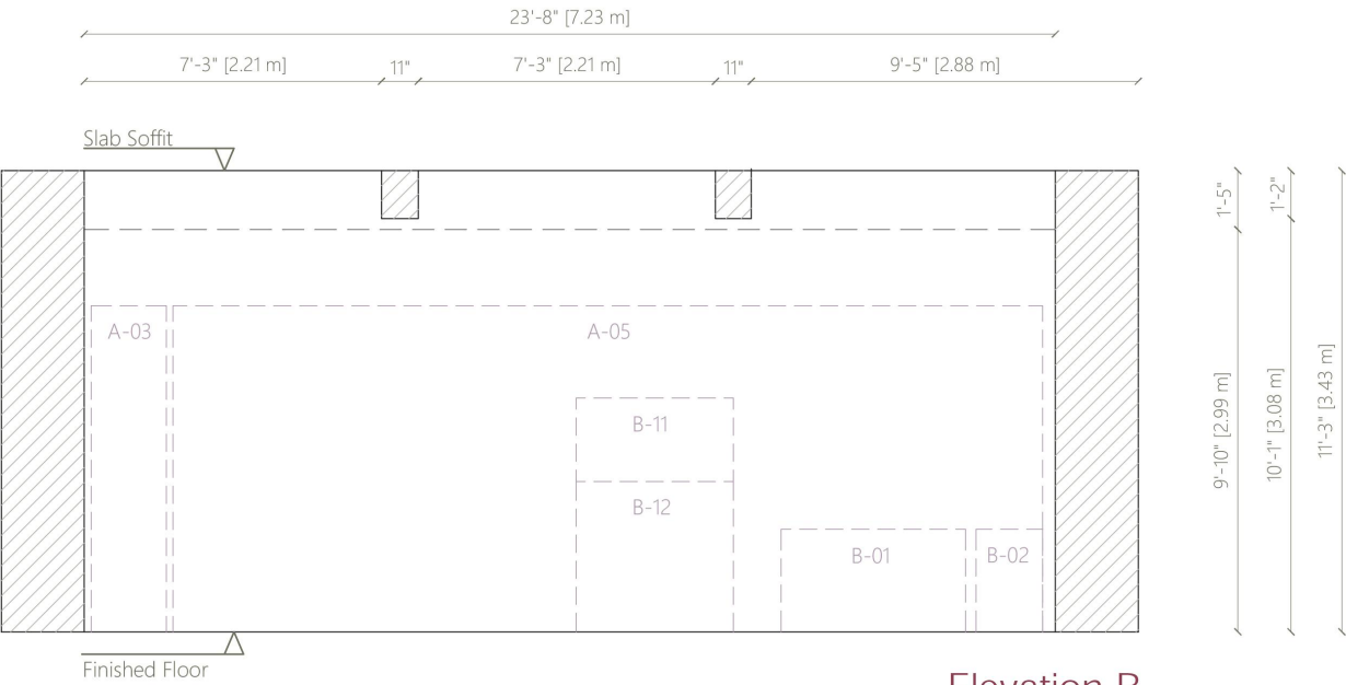
Elevation B
