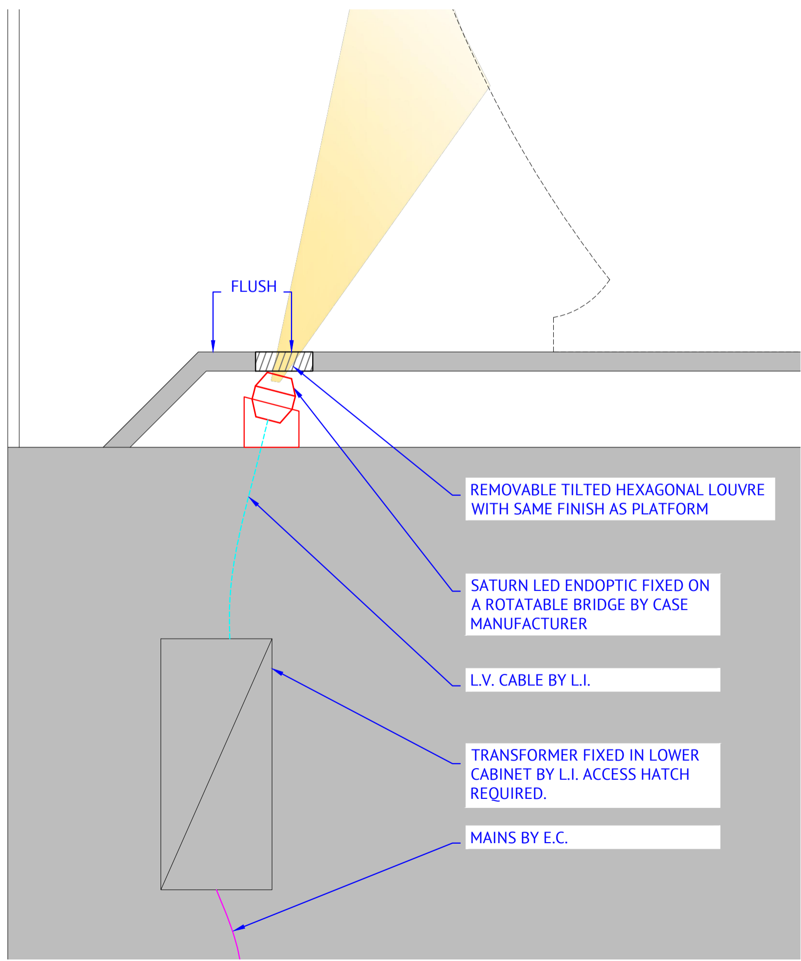
4 SECTION 1:2
